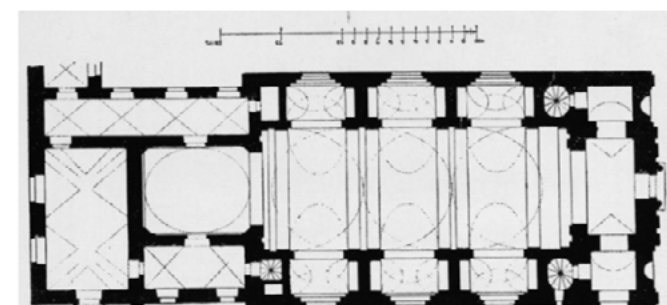
(Obr. 11) Půdorys kostela
